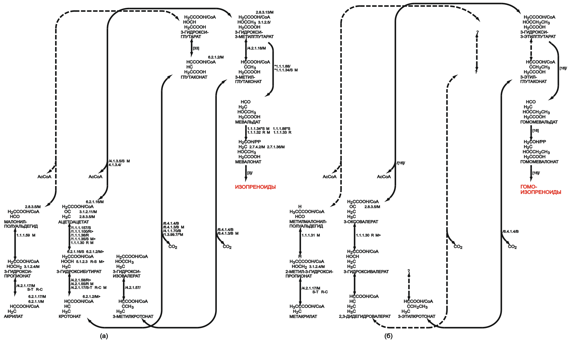
Рис. 5. Периодические последовательности биосинтеза изопреноидов (а) и гомоизопреноидов (б).
